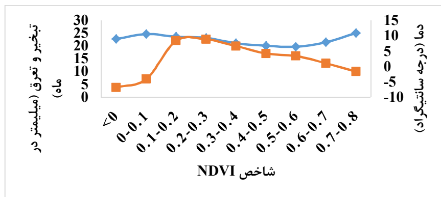
شکل ۴: تغییرات تبخیر و تعرق در ارتباط با دما در دامنه‌های مختلف پوشش گیاهی ماه ژانویه‌ی سال ۲۰۰۸ Figure4: changes of evapotranspiration in relation to temperature in different NDVI in January of 2008
