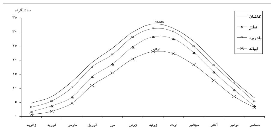
شکل شماره ۱ نمودار تغییرات میانگین دمای ماهانه ایستگاههای منطقه
