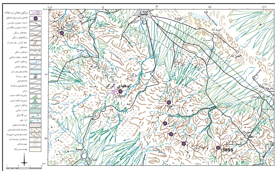
نقشه شماره ۴ ژئومورفولوژی محدوده مورد بررسی و موقعیت سیرکهای مورد مطالعه
