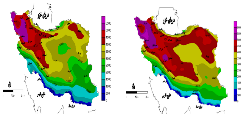
شکل ۲ میانگین مجموع درجه ساعت نیاز گرمایشی ژانویه طی دوره ۲۰۱۵-۲۰۵۰ تحت سناریو A1B
