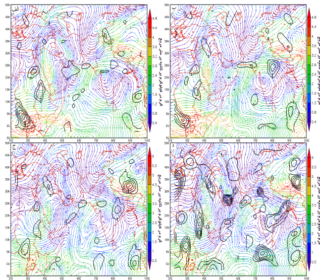
شکل ۷ همگرایی جریان رطوبت جو در طی توفان فت بر روی چابهار در تراز ۵۰۰ هکتوپاسکال برای ساعات‌های الف: ۳/۳۰، ب: ۹/۳۰، ج: ۱۵/۳۰ و د: ۲۱/۳۰ روز ۱۴ خرداد ۱۳۸۹ (منحنی میزان همگرایی رطوبت را براساس گرم بر کیلوگرم بر متر مربع در ثانیه نشان می‌دهد).
