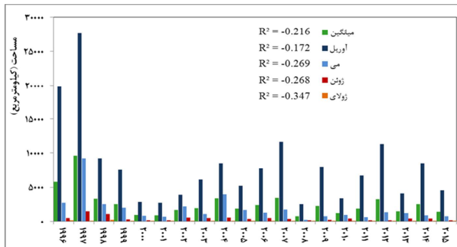
شکل ۳: نمودار میزان تغییرات ماهانه مساحت پوشش برفی در دوره ۱۹۹۶ تا ۲۰۱۵
