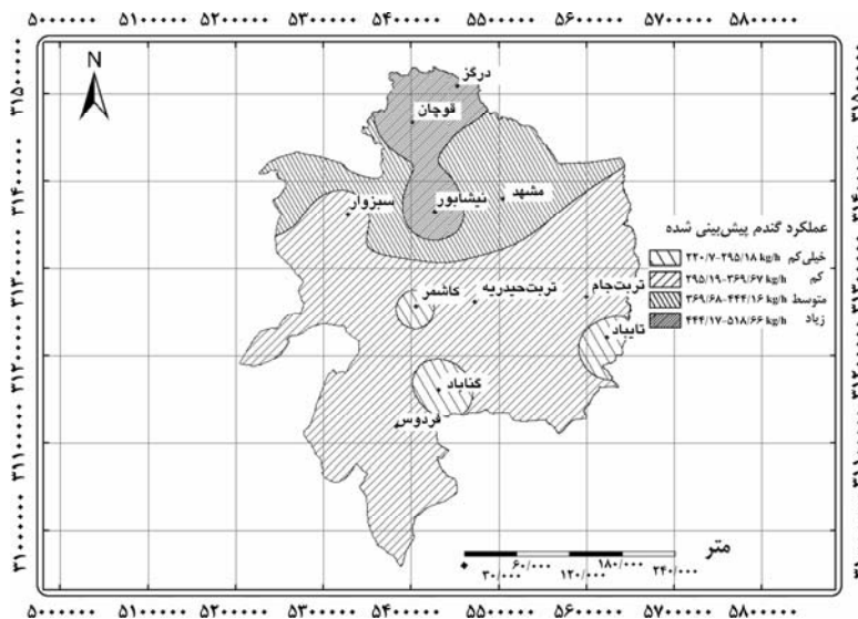
شکل ۳ میانگین فضایی عملکرد گندم دیم محاسباتی در سطح منطقه
