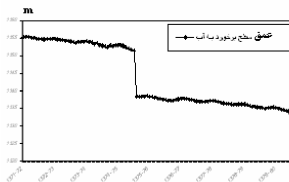
شکل ۲ هیدروگراف آب زیرزمینی دشت نیشابور طی دوره آماری ۱۳۷۱ تا ۱۳۸۰
