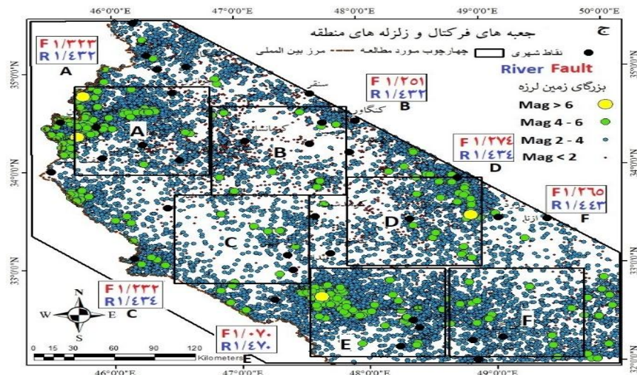
شکل ۹. رابطه بین مقادیر میانگین ارزش فازی و بُعد فرکتالی گسل‌ها (الف)، همپوشانی جعبه‌های بررسی فرکتالی با نتایج مدل فازی (ب) و کانون‌های زلزله (ج)
