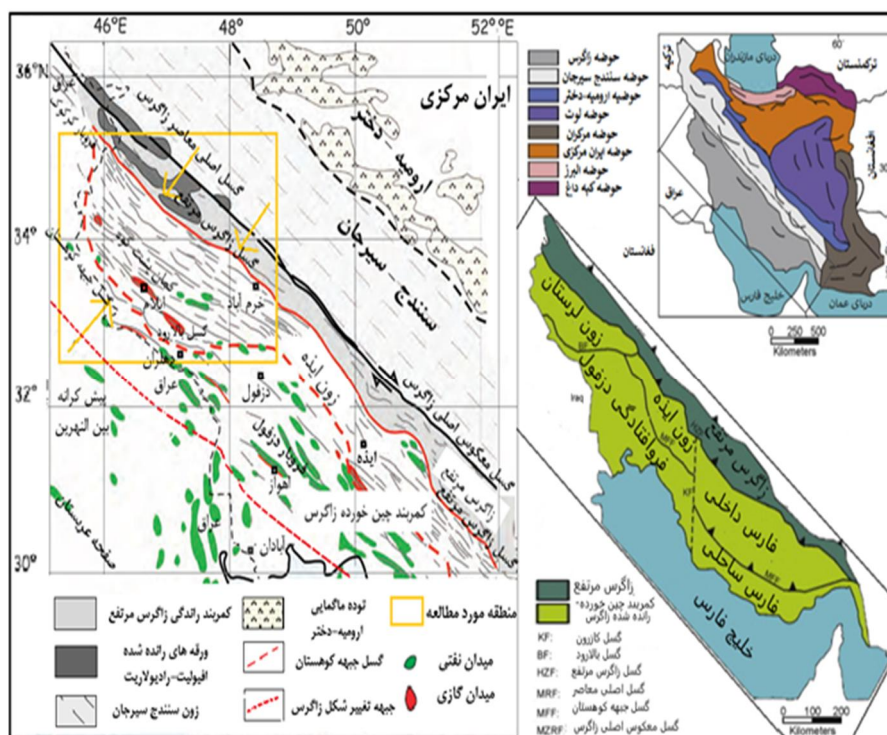
شکل ۱: موقعیت جغرافیایی منطقه مطالعاتی برگرفته از (صحرانیان و همکاران، ۲۰۱۵: ۱۰۵؛ ورگس و همکاران، ۲۰۱۱: ۷۴)
