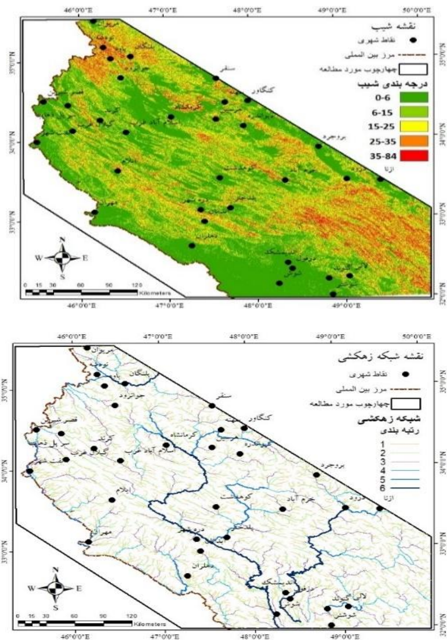
شکل ۵: لایه‌های اطلاعاتی اولیه استفاده شده در فرایند تحقیق
