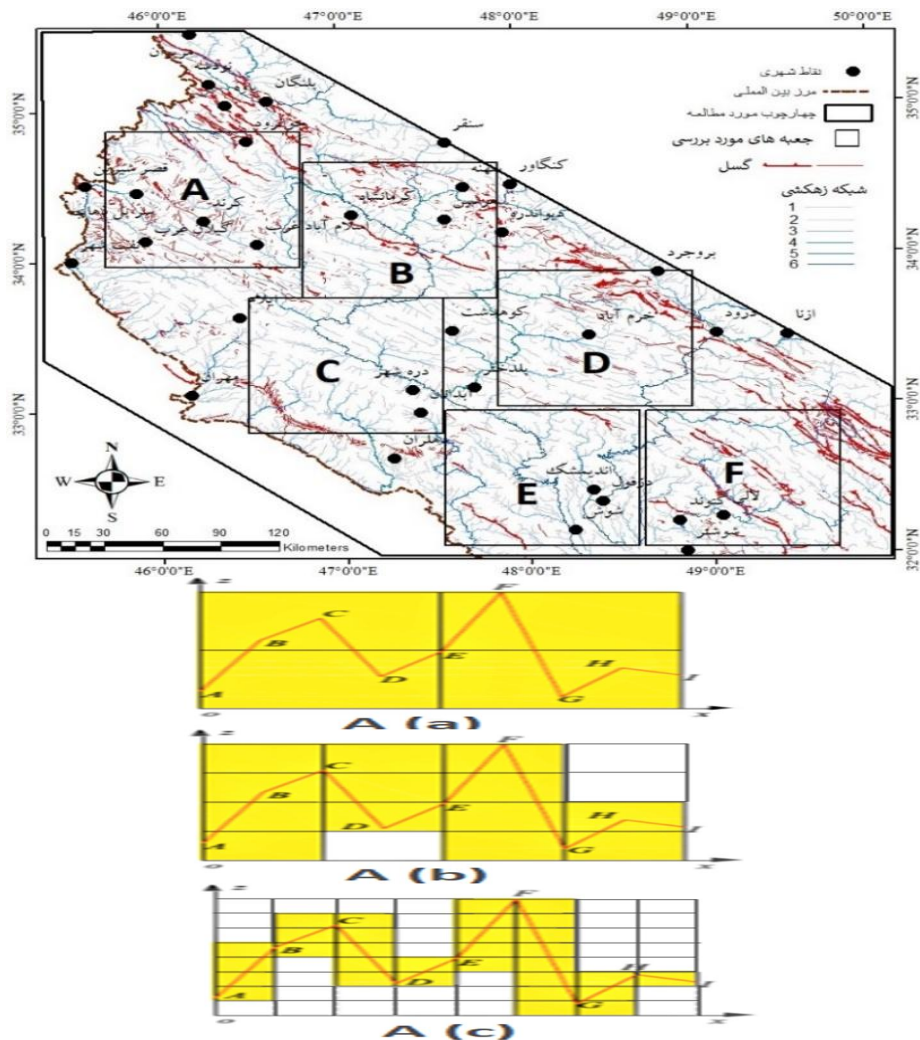
شکل ۲: توزیع جعبه‌های پوشاننده منطقه مطالعاتی و نحوه پوشش عارضه با جعبه‌ها (برای مثال جعبه A در اندازه‌های مختلف تا سه مرتبه تغییر یافته از (آی و همکاران، ۱۴۰۲: ۶۱۳).
