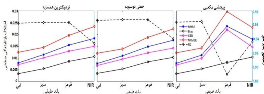
شکل ۳: شاخص‌های آماری مربوط به نتایج روش‌های متفاوت باز نمونه‌گیری برای اختلاف زمانی ۱۶ روزه‌ی سال ۲۰۱۸
