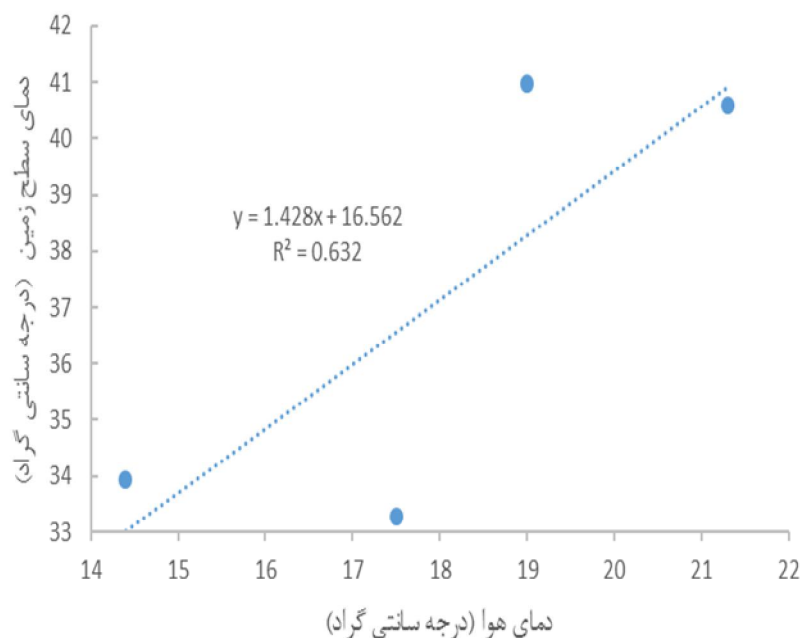
شکل ۱۸: میزان همبستگی دمای سطح زمین و دمای هوا طی سال‌های ۱۳۷۳ تا ۱۳۹۵
