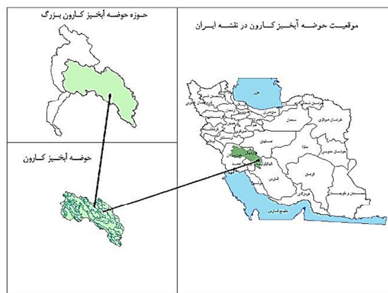
شکل ۱ موقعیت حوضه آبخیز کارون نسبت به حوضه آبخیز کارون بزرگ و کشور ایران
