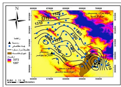
شکل ۳ نقشه سطح آب در سال ۱۳۹۲
