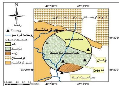
شکل ۹ نقشه حساسیت رسوبات محدوده انتخاب‌شده
