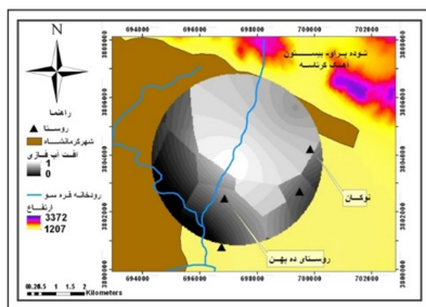
شکل ۷ تعیین عضویت لایه افت سطح آب
