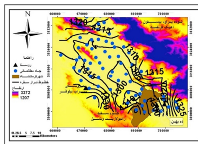
شکل ۲ نقشه سطح آب در سال ۱۳۷۰
