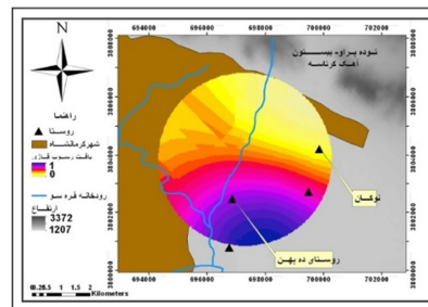
شکل ۶ تعیین عضویت لایه بافت رسوبات
