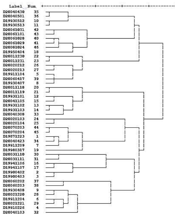
شکل ۲ نمودار خوشه‌بندی براساس ۳ عامل و ۴۶ روز بارش فوق‌سنگین غرب و جنوب غرب حوضه آب‌خیز دریاچه ارومیه
