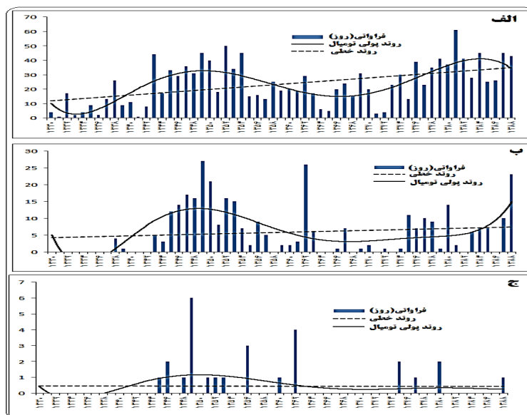
شکل ۳ خط روند خطی و پلی نومیال درجه ۶ فراوانی سالانه روزهای فرین گرم الف- روزهای گرم، ب- روزهای بسیار گرم، ج- روزهای ابرگرم
