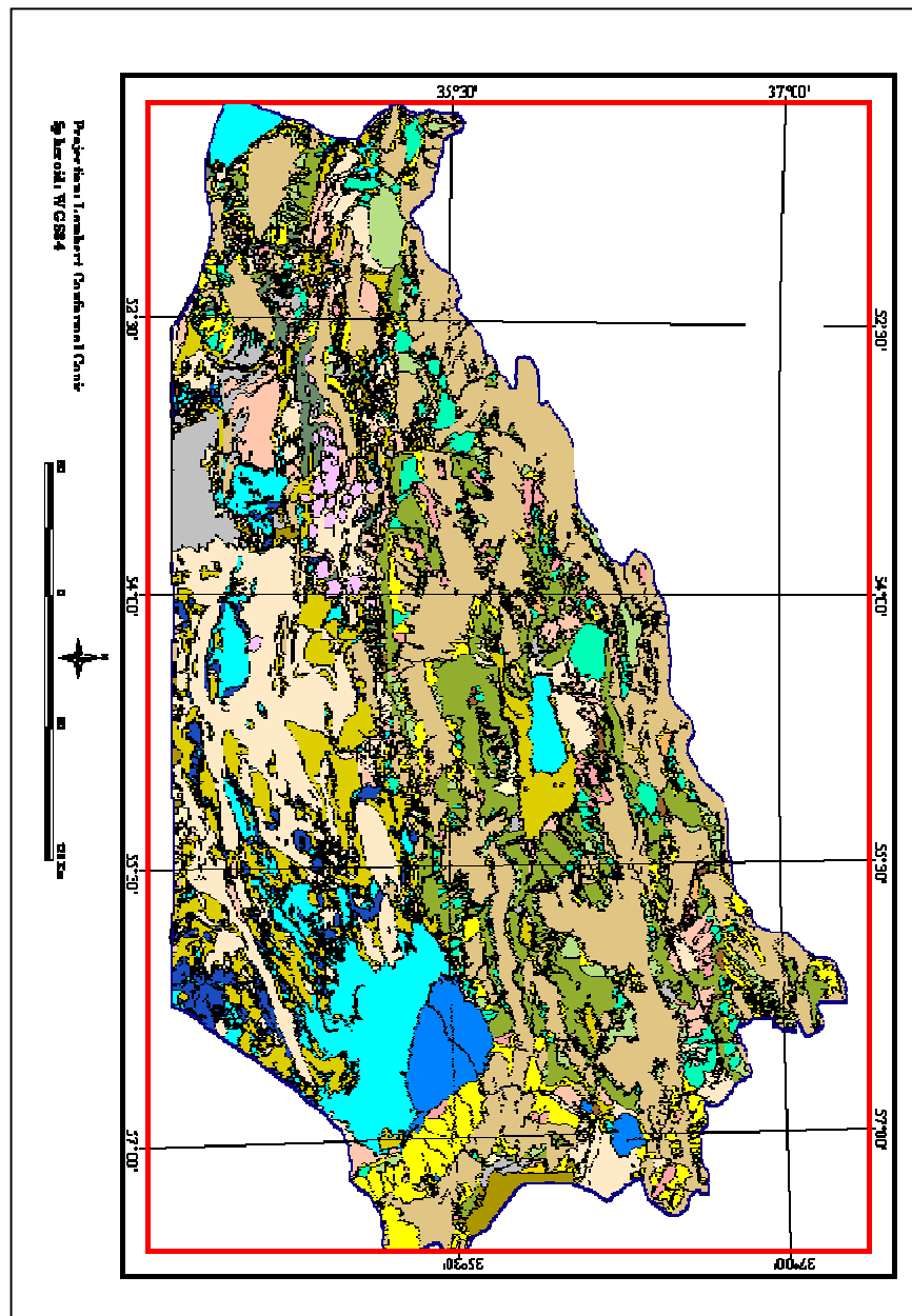
شکل 6 واحدهای زمینشناسی استخراج شده در نرم افزار Arc View 3/2a
