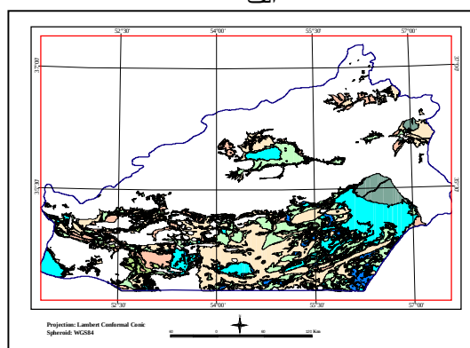
شکل 23 الف- مجموع مناطق مساعد برای کشاورزی و زیستی؛ ب- مجموع پلایاها در استان سمنان که بدون شرایط زیستی است
