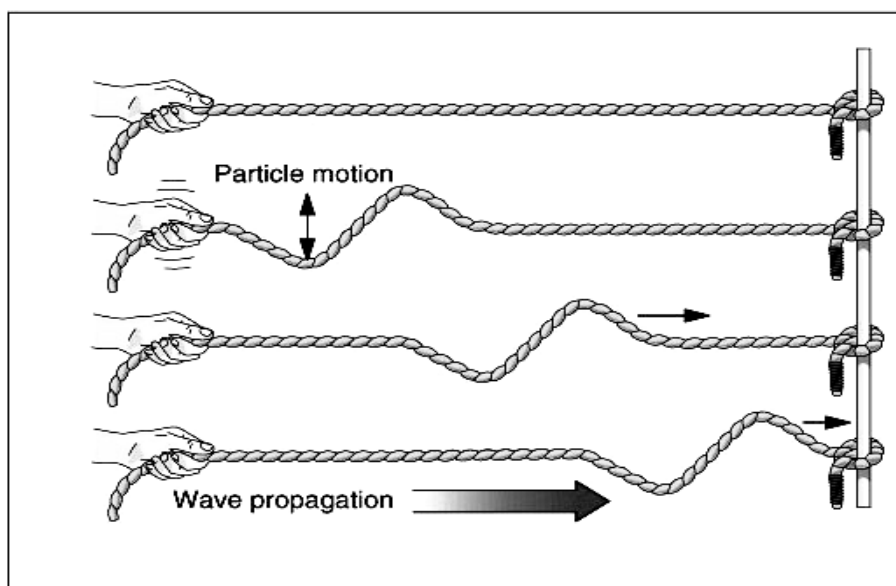
شکل ۲ امواج در لایه‌های زمین و جایگزینی مکان و زمان در یک دید فضایی
