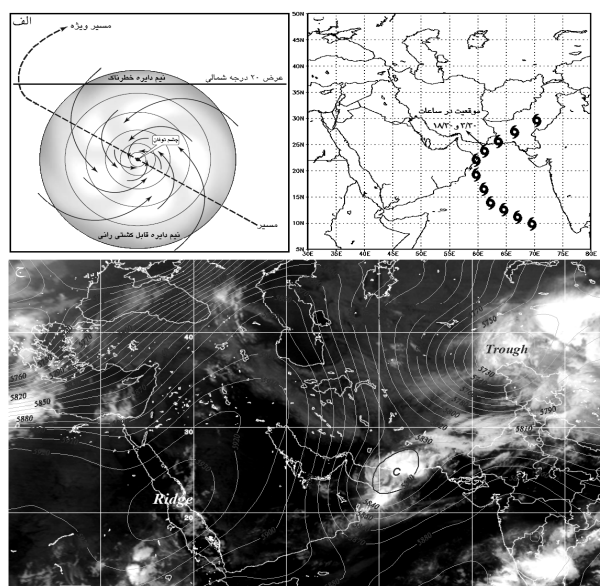
شکل ۲ الف: ساختار و شمای کلی یک توفان حاره ای نمونه از دیدگاه مخاطرات جوی از آلابی، ۲۰۰۷: ۴۹۲؛ ب: مسیر واقعی توفان فت از بدو تشکیل تا روز انهدام و موقعیت آن بر روی چابهار از روز ۱ تا ۷ ژوئن ۲۰۱۰؛ ج: تصویر ترکیبی مادون قرمز ماهواره متوست ۹ و آرایش توپوگرافی ارتفاع ژئوپتانسیل تراز ۵۰۰ هکتوپاسکال در ساعت ۱۵/۳۰ روز ۵ ژوئن ۲۰۱۰
