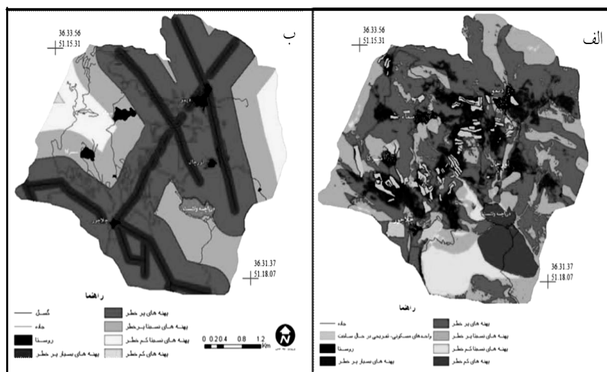
شکل ۳ پهنه‌بندی نواحی پرخطر، الف: مخاطره لغرشی؛ ب: مخاطرات لرزشی
