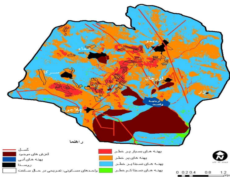
شکل ۴ نقشه پهنه‌بندی مخاطرات زمین در محدوده مطالعه شده
