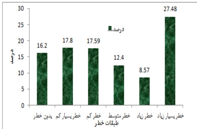
شکل ۱۳ پهنه‌بندی خطر فرسایش خندقی در حوضه آبریز دیره
