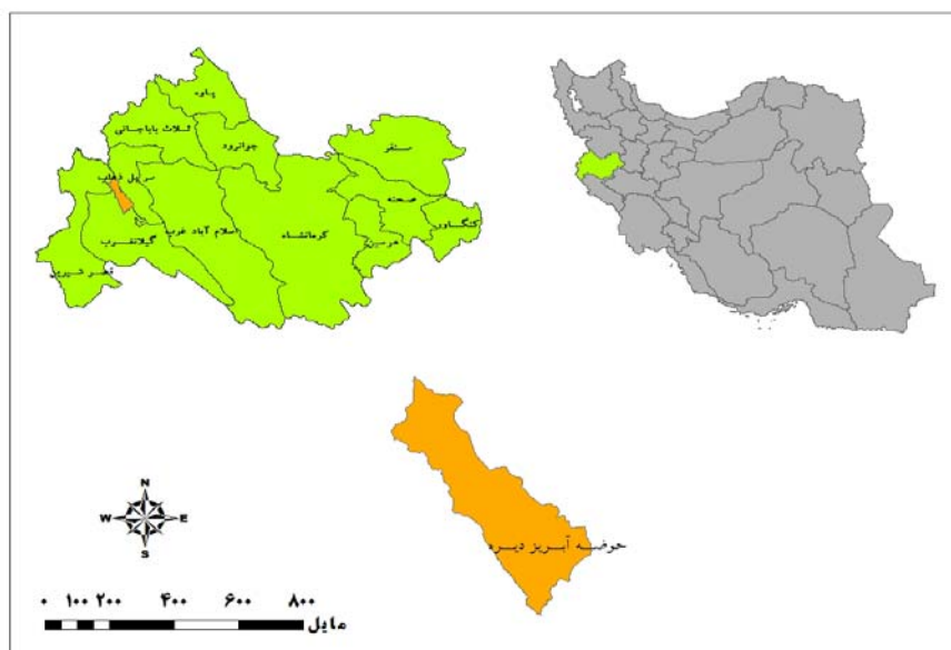
شکل ۲ نقشه محدوده مورد مطالعه
