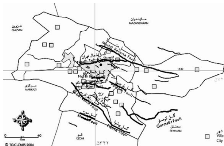
شکل ۱ نقشه پراکنش گسل‌ها نسبت به شهر تهران [۱۰]
