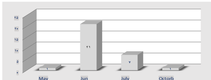
شکل ۲ فراوانی ماهانه توفان‌های حاره‌ای مؤثر بر سواحل جنوبی ایران (۲۰۱۵-۱۸۷۱)
