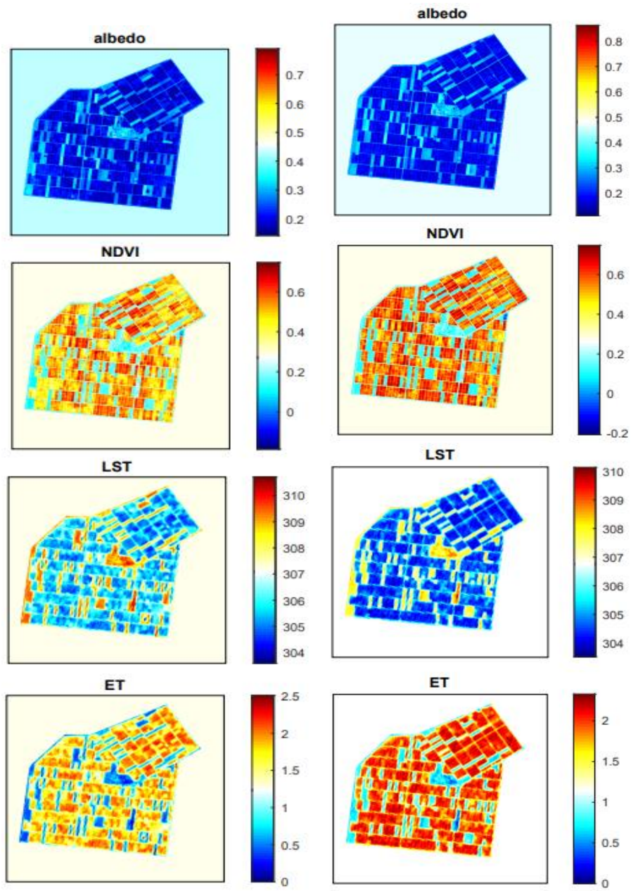
شکل ۷- توزیع مکانی آلبدو، شاخص پوشش گیاهی، دمای سطحی و تبخیر- تعرق واقعی لحظه‌ای حاصل ریزمقیاس نمایی (چپ) و حاصل تصویر واقعی لندست (راست)
