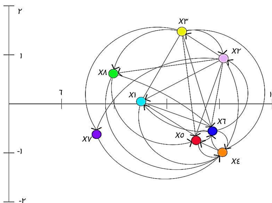
شکل: تحلیل روابط علت و معلولی عوامل تأثیرگذار بر احساس امنیت شهری در کلانشهر تهران از دیدگاه خبرگان
