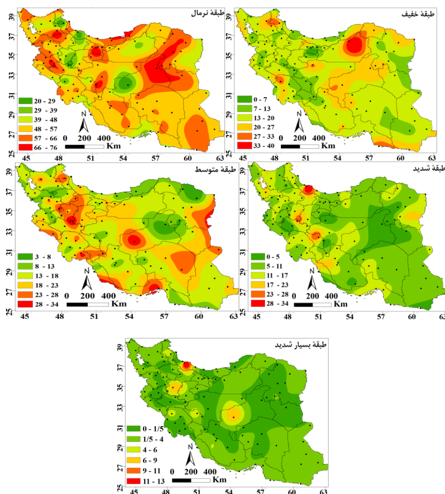
شکل ۴: شاخص خشکسالی خودتنظیم پالمر (SC-PDSI)
