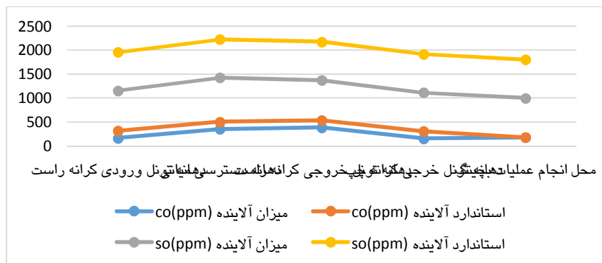
شکل ۱: نتایج اندازه‌گیری میزان SO 2 و CO ایستگاه‌های منتخب سد
