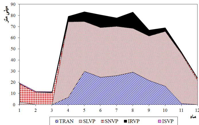
شکل ۷ مؤلفه‌های تبخیر شبیه‌سازی شده حوضه معرف کسلیان (۱۹۹۲)
