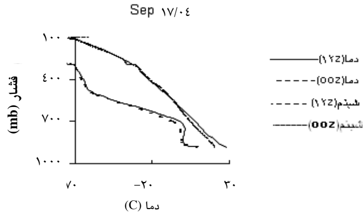
شکل ۲ نمودارهای skew-T رادیوساوند مربوط به تاریخ ۱۷ سپتامبر ۲۰۰۲ در دو زمان صفر و ۱۲:۰۰ به وقت گرینویچ
