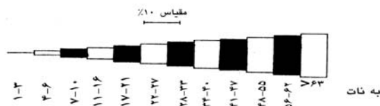
شکل ۱ گلبادهای سطح زمین ایستگاه‌های سینوپتیک یزد در ماه‌های مختلف سال [۲۳].
