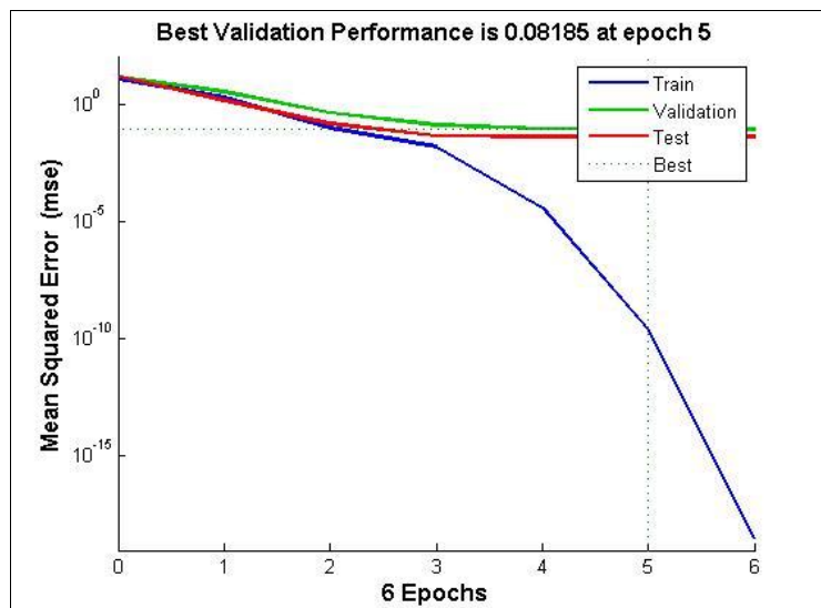
شکل 7 برازش تعداد دفعات تکرار در شبکهٔ عصبی
