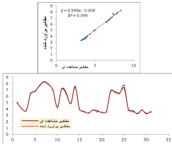
شکل 10 مقادیر مشاهده‌ای و برآوردشده به متر در ANN2
