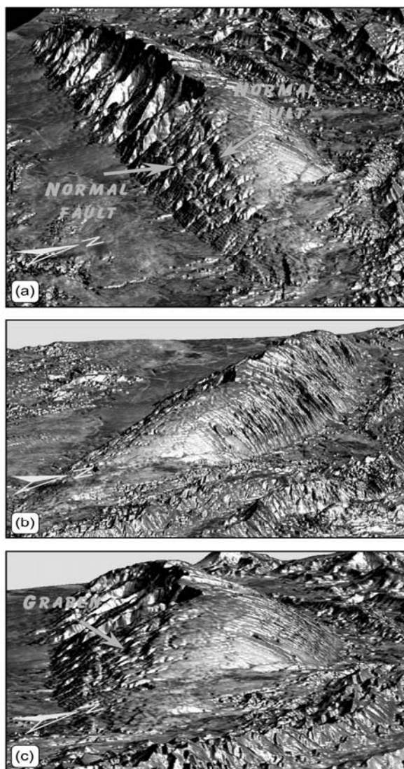
شکل ۱۳ سه نمای جزئی از سیمای نگرشکی در ناحیه پلانژ جنوب خاوری تاقدیس کوه آسماری در مدل سه‌بعدی ASTER. این نماها، با تغییر زوایای ارتفاع و آزیموت نقطه دید، در محیط نرم‌افزار ۶/۴ ER Mapper ایجاد شده‌است. چنانکه ملاحظه می‌شود، در ناحیه ستیغ مجاور با یال جنوب باختری تاقدیس، عملکرد گسل‌های عادی (با فرایند NW-SE) باعث شکل‌گیری یک ساختار فروزمین (Graben) شده‌است.
