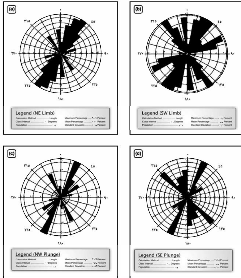
شکل ۱۸ نمودارهای توزیع طول تجمعی شکستگیها در قلمروهای ساختاری تاقدیس کوه آسماری (همچنین، نگاه کنید به شکل‌های ۱۷ و ۱۹).
