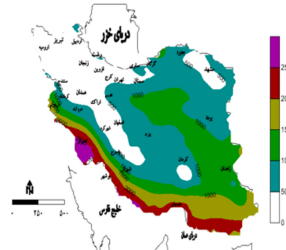
شکل ۱۵ میانگین مجموع درجه ساعت نیاز سرمایشی اوت طی دوره ۲۰۱۵-۲۰۵۰ تحت سناریو AIB
