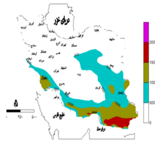
شکل ۱۱ میانگین مجموع درجه ساعت نیاز سرمایه‌اشی آوریل طی دوره ۲۰۱۵-۲۰۵۰ تحت سناریو A1B
