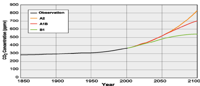
نمودار ۱ میزان روند تغییرات میزان دی‌اکسیدکربن موجود در جو در دوره زمانی ۲۱۰۰-۱۸۵۰
