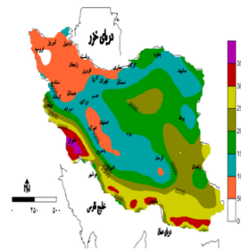
شکل ۱۳ میانگین مجموع درجه ساعت نیاز سرمایه‌اشی ژوئن طی دوره ۲۰۱۵-۲۰۵۰ تحت سناریو A1B
