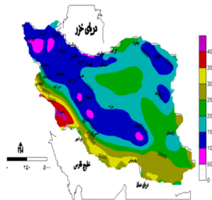
شکل ۱۴ میانگین مجموع درجه ساعت نیاز سرمایه‌اشی ژوئیه طی دوره ۲۰۱۵-۲۰۵۰ تحت سناریو A1B
