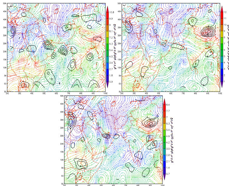
شکل ۶ همگرایی جریان رطوبت جو در طی توفان بر روی چابهار در تراز ۷۰۰ هکتوپاسکال برای ساعت‌های الف: ۳/۳۰، ب: ۲۱/۳۰، ج: تراز ۶۰۰ هکتوپاسکال در ساعت ۲۱/۳۰ روز ۱۴ خرداد ۱۳۸۹ (منحنی میزان همگرایی رطوبت را براساس گرم بر کیلوگرم بر متر مربع در ثانیه نشان می‌دهد).
