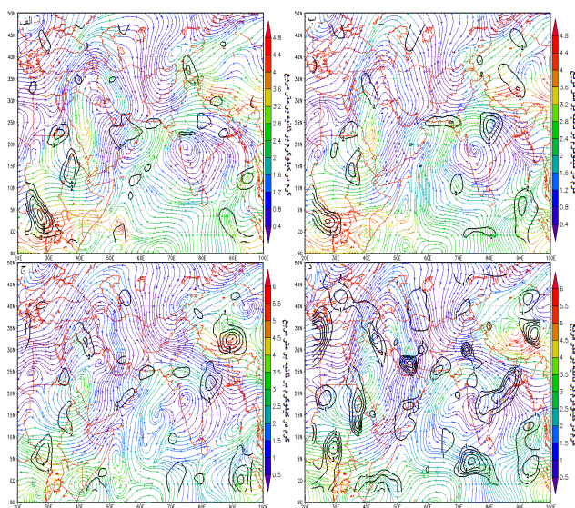
شکل ۷ همگرایی جریان رطوبت جو در طی توفان چابهار در تراز ۵۰۰ هکتوپاسکال برای ساعات‌های الف: ۳/۳۰، ب: ۹/۳۰، ج: ۱۵/۳۰ و د: ۲۱/۳۰ روز ۱۴ خرداد ۱۳۸۹ (منحنی میزان همگرایی رطوبت را براساس گرم بر کیلوگرم بر متر مربع در ثانیه نشان می‌دهد).
