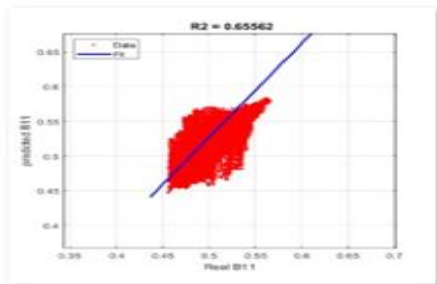
خروجی Regression
