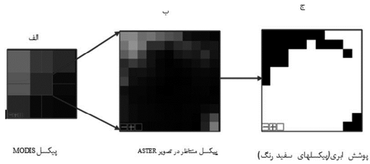
شکل ۶ الف: پیکسل MODIS انتخاب شده؛ ب، ج: جستجو در داخل آن به وسیله ASTER و جداسازی پیکسل‌های پوشش بری از غیر بری
