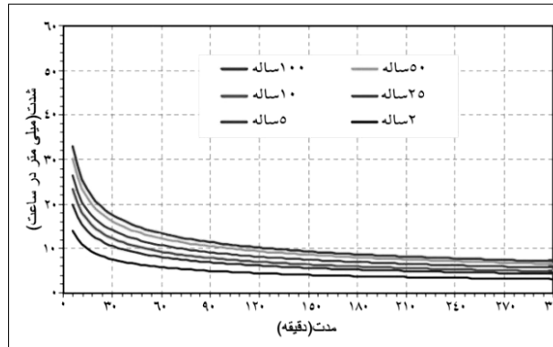
شکل ۸ منحنی شدت، مدت، فراوانی ایستگاه سعداآباد
