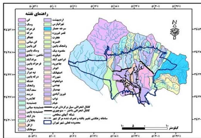
شکل ۳ حوضه‌های زهکشی بعد از توسعه شهر تهران همراه شبکه زهکشی طبیعی و تغییر یافته
