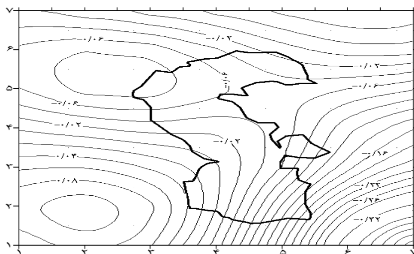
شکل ۴ نقشه مقادیر هم فرارفت دما براساس کل داده‌های لایه‌های جوی ۱۰۰۰ تا ۱۰۰۰۰ هکتوپاسکال در محدوده خزر
