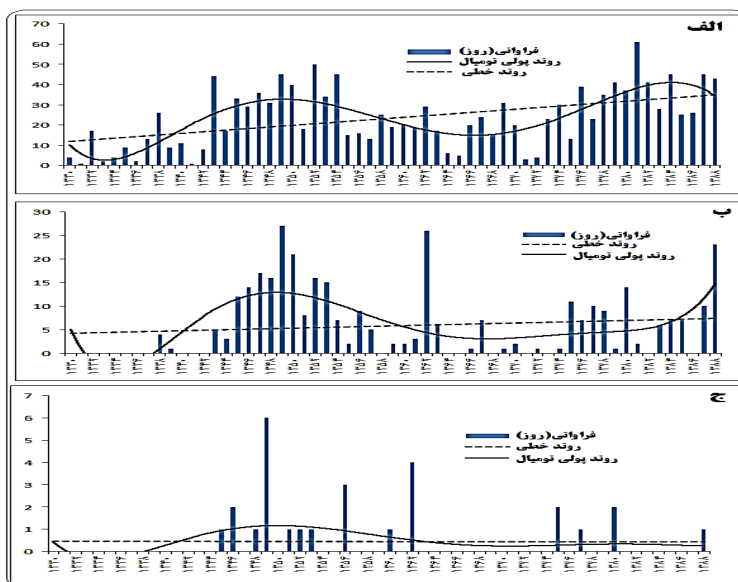
شکل ۳ خط روند خطی و پولی نومیال درجه ۶ فراوانی سالانه روزهای فرین گرم الف- روزهای گرم، ب- روزهای بسیار گرم، ج- روزهای ابرگرم
