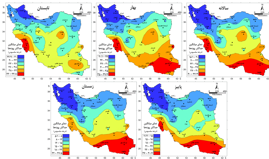
شکل 5 پهنه‌بندی ایران بر مبنای دماهای میانگین حداکثر سالیانه و فصلی (1964-2008م)
