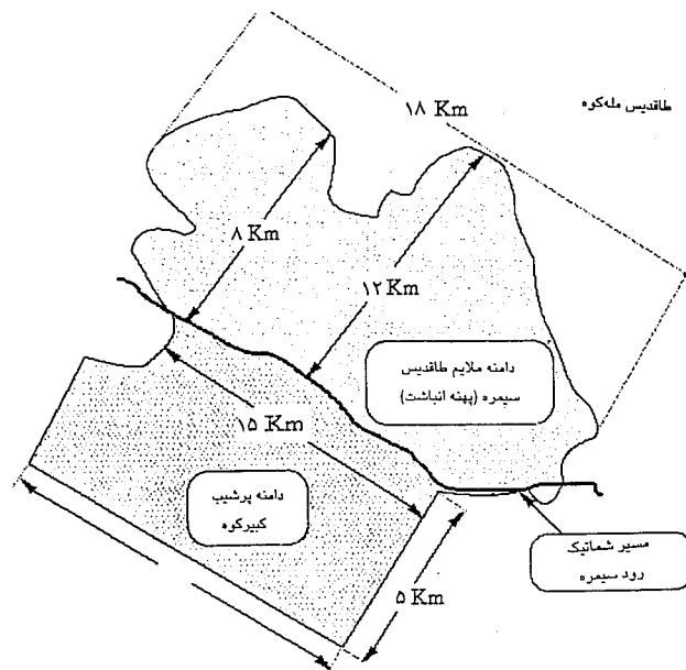
شکل ۳ طرح افقی لغزش در منطقه سیمره [۲]
