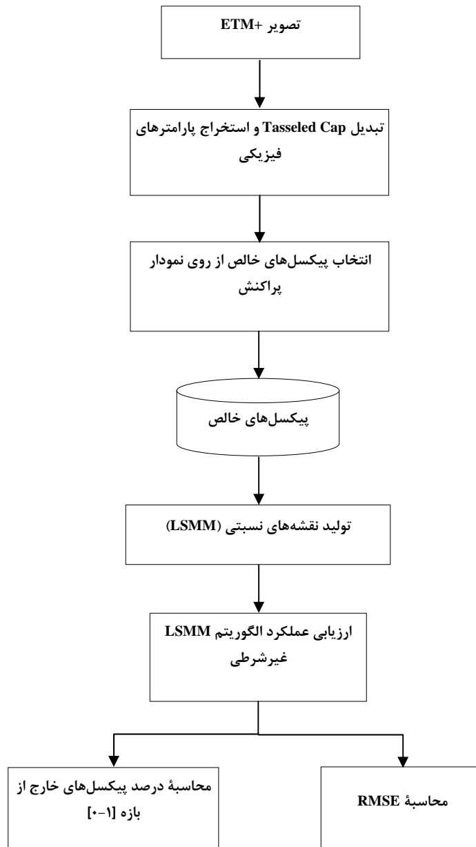
شکل ۴ روش پیشنهادی برای استخراج پیکسل‌های خالص جهت ورود به الگوریتم LSMM
